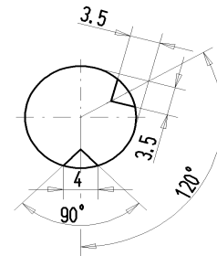
Detail Z:1
